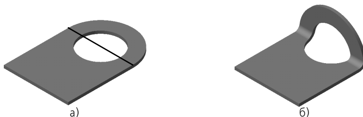
Рис. 97.21. Сгиб детали с отверстием: а) положение линии сгиба, б) результат построения
