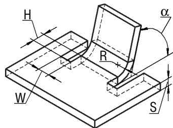
Рис. 95.3. Параметры листовой детали
