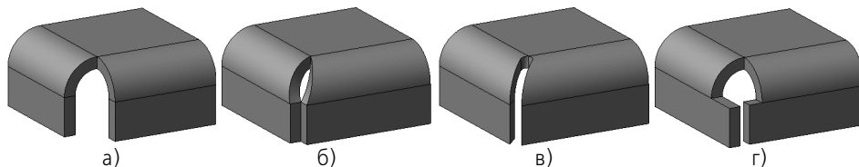
Рис. 97.29. Замыкание угла: а) исходное состояние детали, б), в), г) варианты замыкания угла
