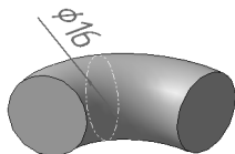
Рис. 117.12. Пример простановки диаметрального размера к грани тороидальной формы В качестве объекта фиксации (см. раздел 117.5.1 на с. 342) может быть выбран точечный объект или плоский объект, перпендикулярный круговой оси тора.
