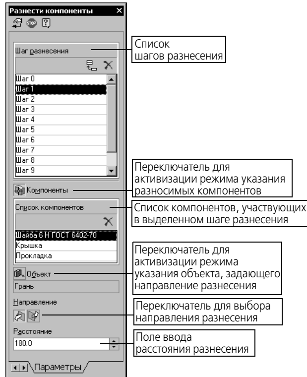
Рис. 124.1. Задание параметров разнесения компонентов
