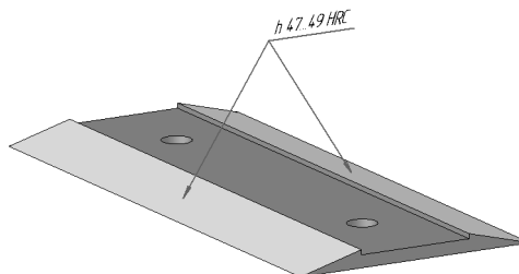
Рис. 118.5. Пример простановки линии-выноски
