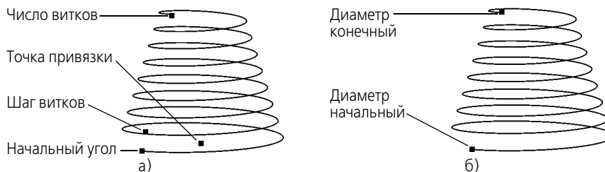
Рис. 94.1. Характерные точки конической спирали:
