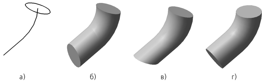
Рис. 87.6. Кинематический элемент: а) эскизы сечения и траектории, б) перемещение сечения с сохранением угла наклона, в) перемещение сечения параллельно самому себе, г) перемещение сечения ортогонально траектории.
