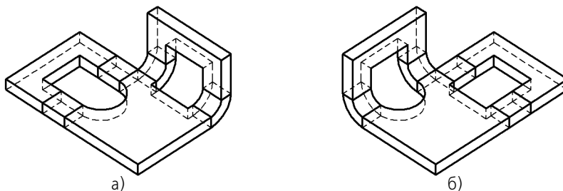
Рис. 99.7. Вырезы, построенные способом На глубину : а) вид детали сразу после создания вырезов, б) результат изменения состояния сгибов
