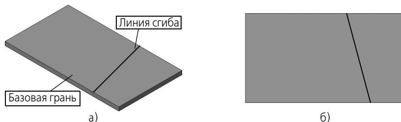
Рис. 97.28. Исходный элемент подсечки: а) изометрическая проекция, б) проекция исходного элемента на базовую грань
