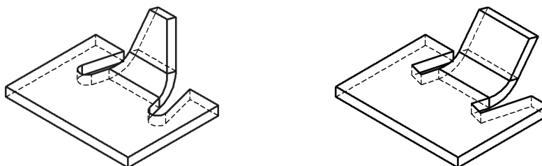
Рис. 97.18. Освобождение сгиба при отличном от нуля угле на сгибе
