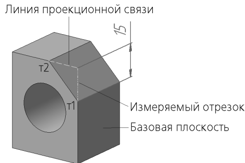
Рис. 117.2. Пример простановки линейного размера
