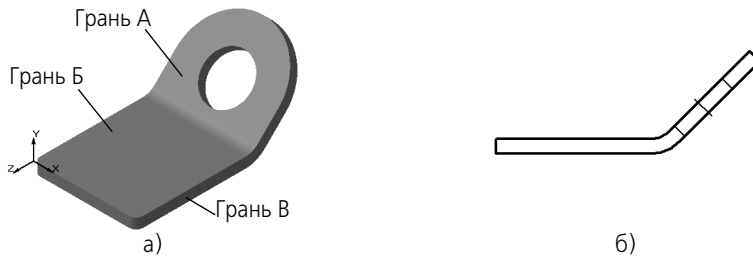
Рис. 100.8. Листовая деталь: а) в проекции Изометрия XYZ , б) главный вид
