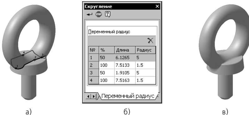
Рис. 91.4. Построение скругления с переменным радиусом: а) указание точек, б) задание параметров скругления, в) результат выполнения команды
