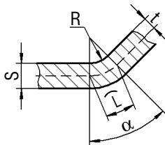
Рис. 95.10. Сечение сгиба плоскостью, перпендикулярной линии сгиба (нейтральная линия показана штрихами)
