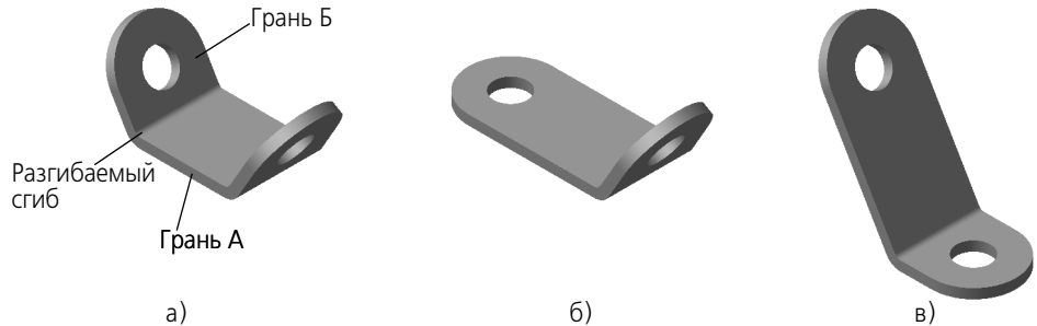
Рис. 100.1. Зависимость результата разгибания от выбора неподвижной грани: а) исходное состояние детали, б) неподвижна грань А, в) неподвижна грань Б
