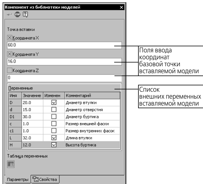
Рис. 131.1. Панель свойств при вставке библиотечной модели
