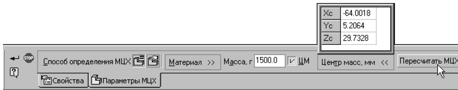
Рис. 85.15. Расчет МЦХ по массе
