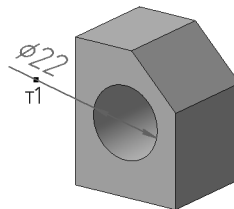
Рис. 117.9. Диаметральный размер с ручным размещением размерной линии
