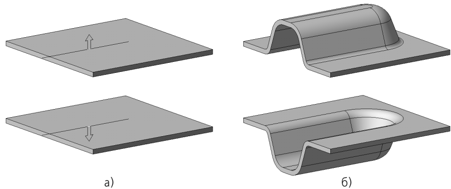
Рис. 101.2. Направление построения штамповочного элемента: а) выбор направления, б) результат построения
