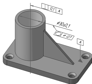
Рис. 118.8. Пример простановки допуска формы и расположения поверхности
