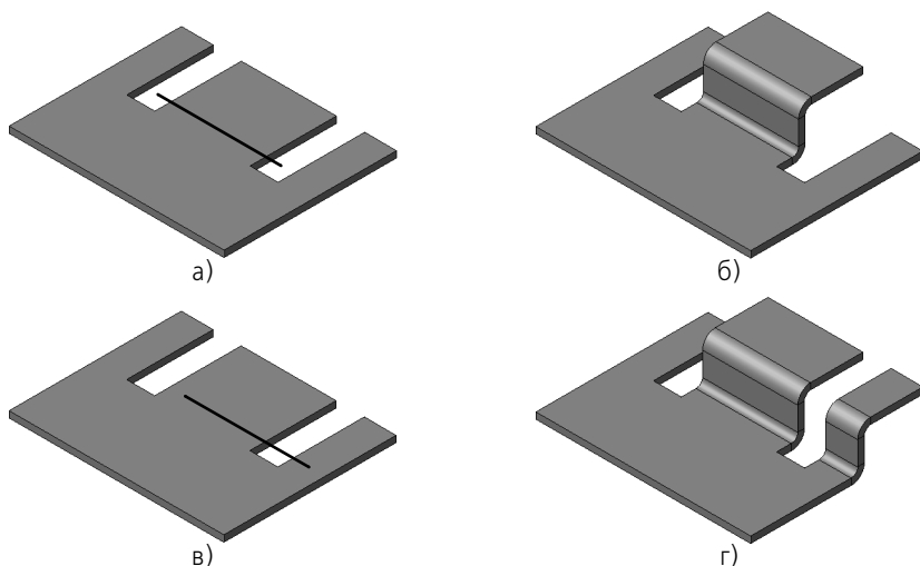
Рис. 97.24. Зависимость результата построения подсечки от положения линии сгиба: а), в) варианты положения линии сгиба, б), г) соответствующие результаты выполнения операции
