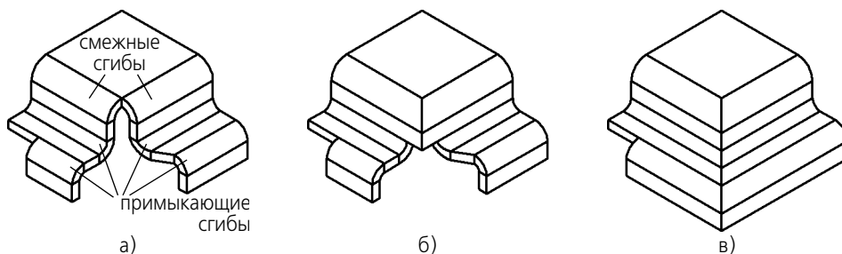
Рис. 97.33. Замыкание сгиба: а) исходное состояние детали, б) замыкание без продолжения, в) замыкание с продолжением
