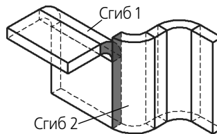
Рис. 97.5. Пример расположения сгибов, позволяющего применить освобождение угла: плоская кольцевая грань создаваемого Сгиба 1 частично совпадает с плоской прямоугольной гранью соседнего с ним Сгиба 2
