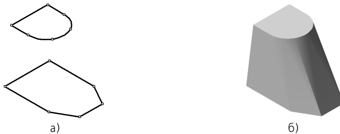
Рис. 87.11. Дуга в верхнем сечении разбита на три сопрягающихся части. В результате контур в сечении не изменился, а результат построения стал предсказуемым
