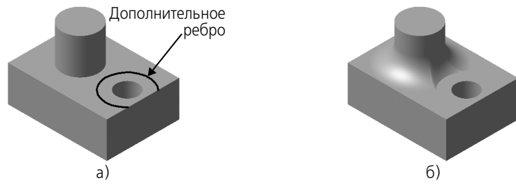
Рис. 104.1. Использование дополнительного ребра: а) исходное состояние детали, б) результат выполнения операции скругления с сохранением кромки
