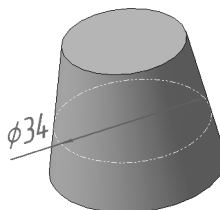
Рис. 117.10. Пример простановки диаметрального размера к грани конической формы
