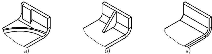
Рис. 100.6. Примеры формообразующих и конструктивных элементов, делающих невозможным разгибание сгиба: а) приклеенный и вырезанный элементы, б) ребро жесткости, в) фаска
