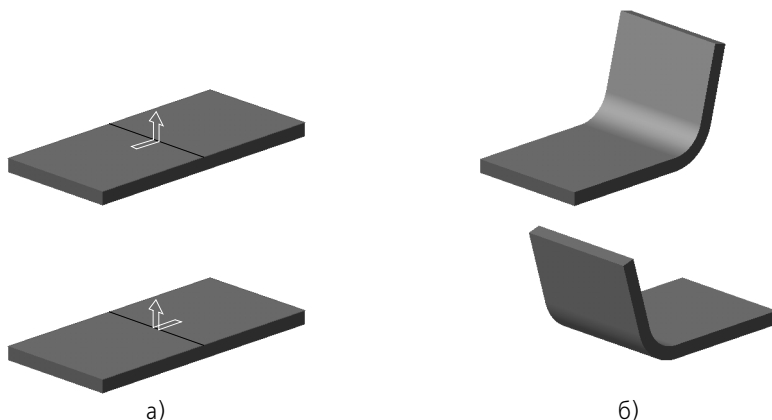
Рис. 97.23. Сгиб по линии: а) направление и неподвижная сторона, б) результат операции
