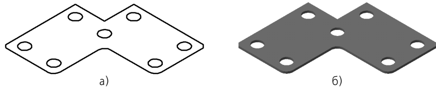
Рис. 96.1. Построение листового тела на основе замкнутого эскиза: а) эскиз, б) листовое тело
