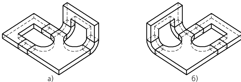
Рис. 99.6. Вырезы, построенные способом По толщине : а) вид детали сразу после создания вырезов, б) результат изменения состояния сгибов
