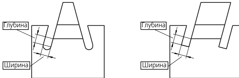
Рис. 97.19. Определение размеров освобождения сгиба при отличном от нуля угле на сгибе
