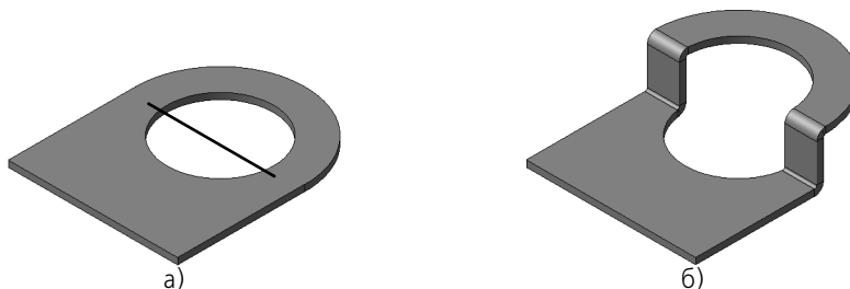
Рис. 97.27. Подсечка в детали с отверстием: а) положение линии сгиба, б) результат построения
