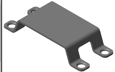
Рис. 95.8. Новые значения переменных и перестроенная деталь
