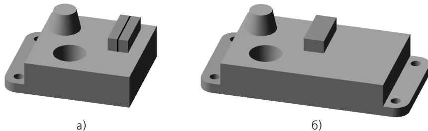
Рис. 93.8. Зеркальное копирование отдельных элементов: а) исходная деталь (плоскость симметрии для копирования показана условно), б) результат копирования основания и лапки относительно средней плоскости прямоугольного выступа
