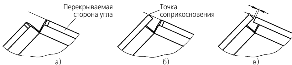
Рис. 97.39. Построение замыкания с перекрытием для тупого угла: а), б) определение положения перекрывающей стороны, в) определение положения перекрываемой стороны
