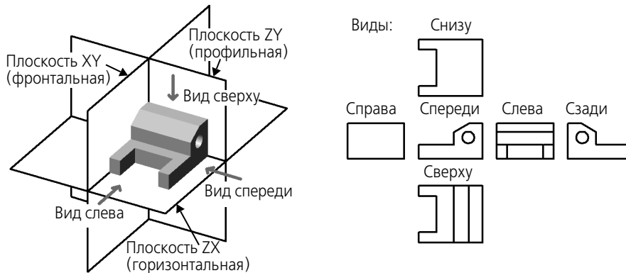
Рис. 88.1. Положение детали относительно координатных плоскостей
