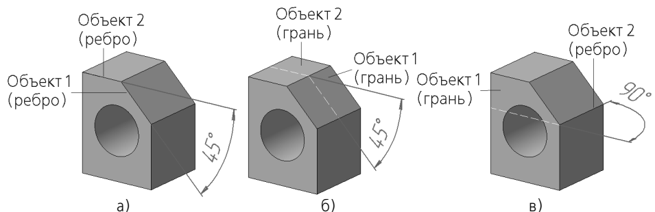
Рис. 117.5. Примеры простановки углового размера: а) между двумя ребрами, б) между двумя гранями, в) между ребром и гранью
