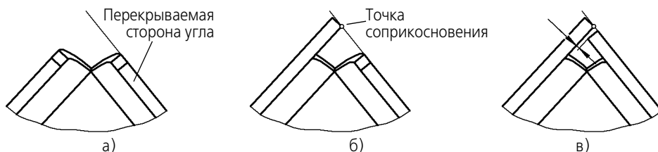
Рис. 97.38. Построение замыкания с перекрытием для острого угла: а), б) определение положения перекрывающей стороны, в) определение положения перекрываемой стороны
