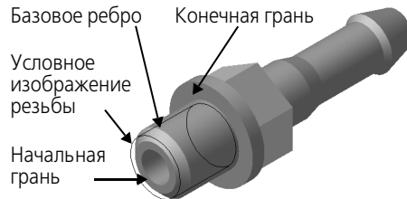
Рис. 119.1. Условное изображение резьбы в детали Ниппель
