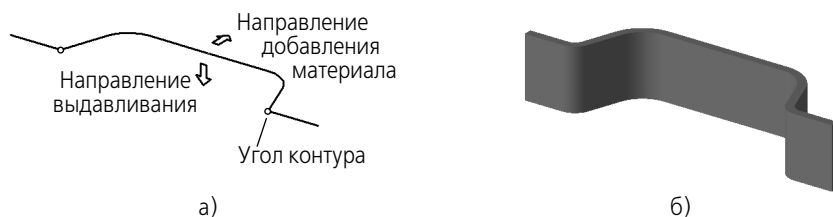
Рис. 96.2. Построение листового тела на основе разомкнутого эскиза: а) эскиз, б) листовое тело
