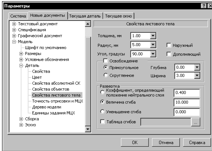
Рис. 95.4. Диалог настройки параметров листового тела для новых деталей
