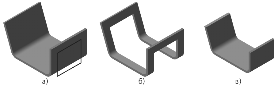
Рис. 99.4. Результат построения выреза в листовых детали:
