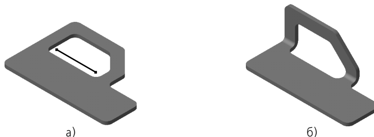
Рис. 97.22. Использование вспомогательной оси в качестве линии сгиба: а) расположение оси, б) результат построения
