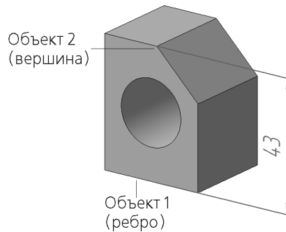
Рис. 117.4. Пример простановки линейного размера от отрезка до точки
