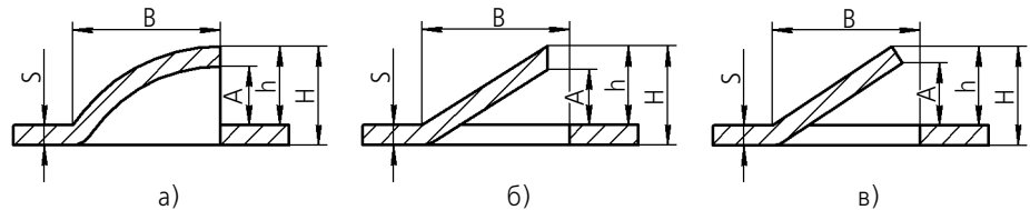
Рис. 101.11. Геометрические параметры жалюзи: а) вытянутых; б) подрезанных с торцом по направлению подрезки; в) подрезанных с торцом по нормали к толщине
