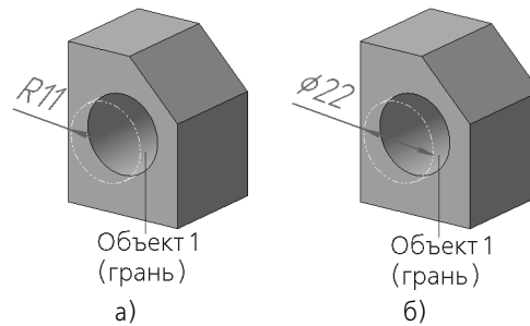
Рис. 117.7. Примеры простановки размеров к грани детали: а) радиального, б) диаметрального
