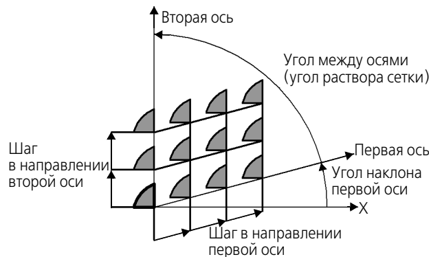
Рис. 93.2. Схема образования параллелограммной сетки
