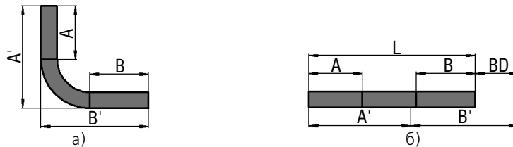
Рис. 95.12. Разгибание сгиба: а) сгиб согнут, б) сгиб разогнут
