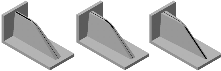
Рис. 91.6. Ребро жесткости с уклоном. Эскиз ребра состоит из трех сегментов. Сегмент, задающий направление уклона, выделен.
