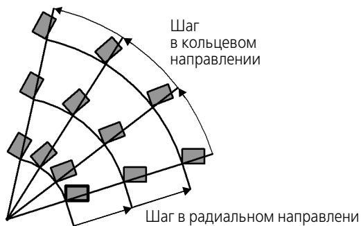
Рис. 93.3. Схема образования концентрической сетки
