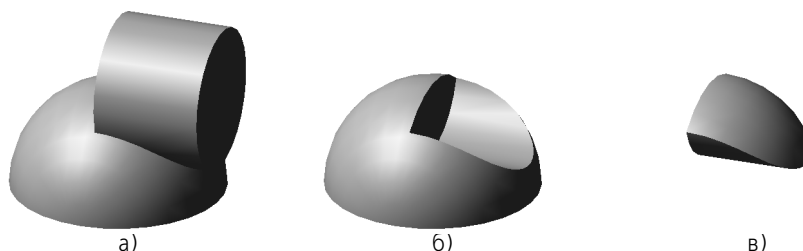
Рис. 89.5. Различные способы вырезания: а) исходные элементы, б) результат вычитания цилиндра из полусферы, в) пересечение цилиндра и полусферы Этот параметр можно задать при вырезании формообразующего элемента любого типа.
