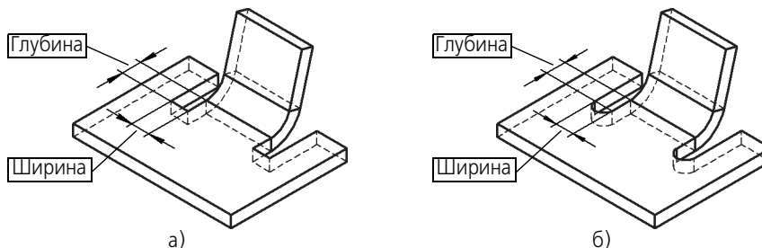
Рис. 97.16. Освобождение сгиба: а) прямоугольное, б) скругленное
