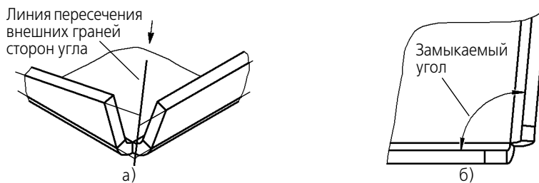
Рис. 97.32. Измерение зазора: а) определение положения плоскости измерения, б) проекция детали на плоскость измерения (вид по стрелке); замыкаемый угол
