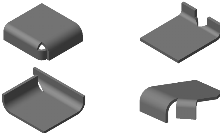
Рис. 97.42. Примеры смежных сгибов, замыкание угла между которыми невозможно
