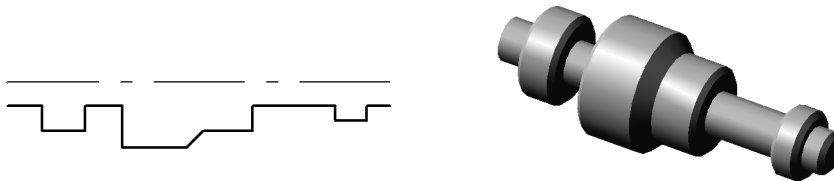
Рис. 87.5. Построение элемента вращения с плоскими торцами
