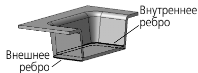
Рис. 101.6. Внутренние и внешние ребра дна штамповки (штамповка рассечена плоскостью, перпендикулярной базовой грани)
