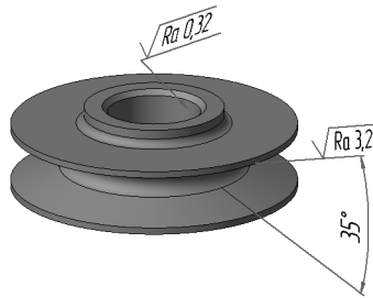
Рис. 118.3. Пример простановки обозначения шероховатости
