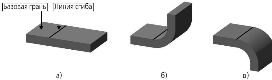
Рис. 97.2. Направление сгиба: а) базовая грань и линия сгиба, б) сгиб в прямом направлении, в) сгиб в обратном направлении
