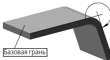
Рис. 97.4. Сгиб в обратном направлении
