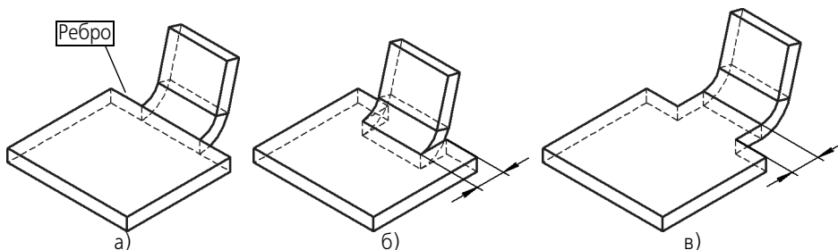
Рис. 97.13. Смещение сгиба: а) нулевое, б) внутрь, в) наружу
