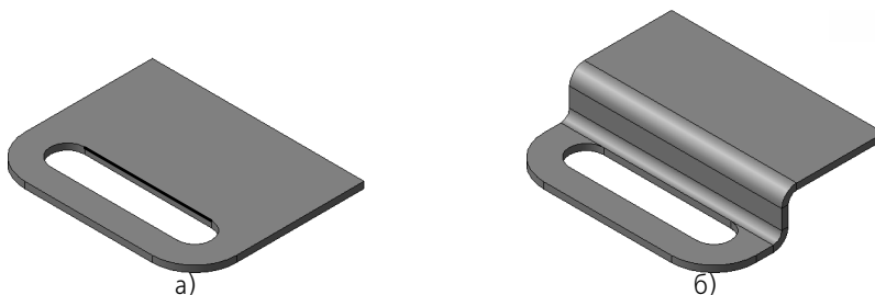
Рис. 97.26. Использование ребра в качестве линии сгиба подсечки: а) расположение ребра, б) результат построения
