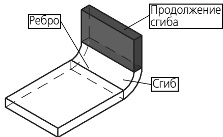
Рис. 97.10. Продолжение сгиба вдоль ребра
