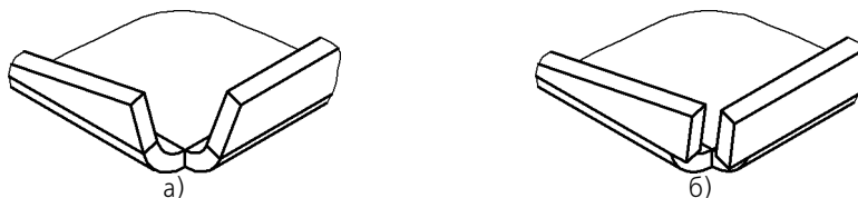
Рис. 97.34. Замыкание встык: а) исходное состояние детали, б) результат замыкания угла (зазор отличен от нуля)
