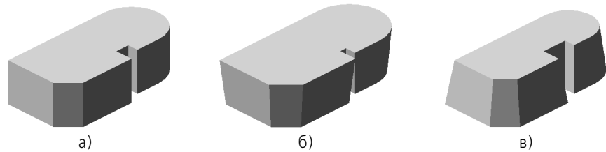
Рис. 87.3. Выдавливание в одном направлении: а) без уклона, б) уклон наружу, в) уклон внутрь
