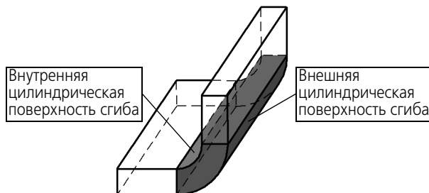
Рис. 97.1. Пример сгиба в листовой детали
