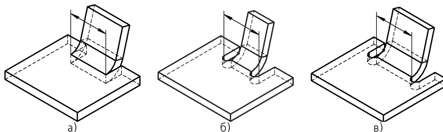
Рис. 97.17. Расположение освобождений: а) ширина сгиба без освобождений, б) освобождения включены в ширину сгиба, в) освобождения не включены в ширину сгиба
