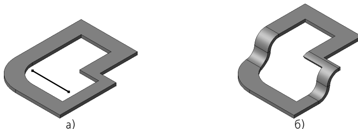
Рис. 97.25. Использование вспомогательной оси в качестве линии сгиба подсечки: а) расположение оси, б) результат построения
