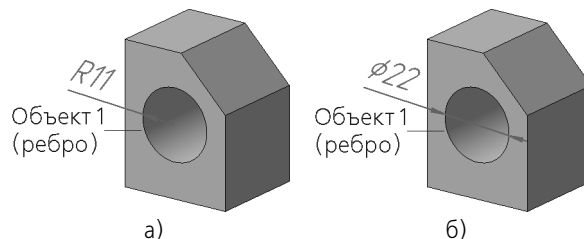
Рис. 117.6. Примеры простановки размеров к ребру детали: а) радиального, б) диаметрального
