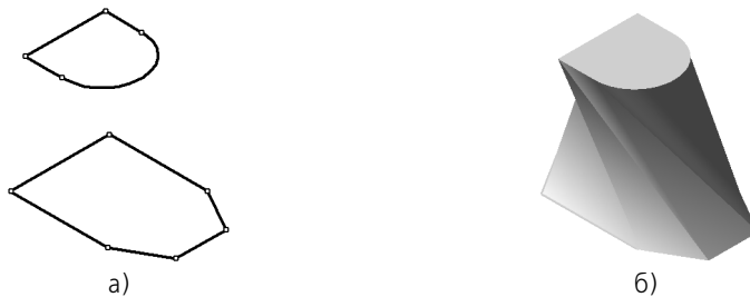
Рис. 87.10. Автоматическое соединение сечений с разной топологией
