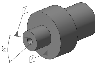
Рис. 118.4. Пример простановки обозначения базы
