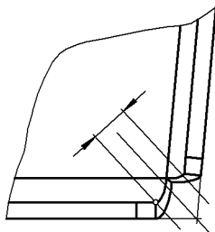
Рис. 97.36. Максимальный зазор при замыкании встык
