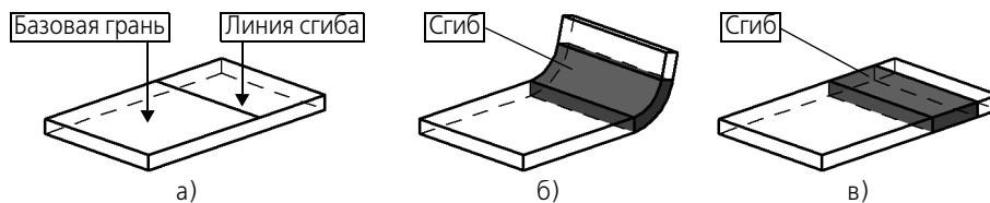
Рис. 97.6. Построение сгиба: а) базовая грань и линия сгиба, б) согнутый сгиб, в) разогнутый сгиб
