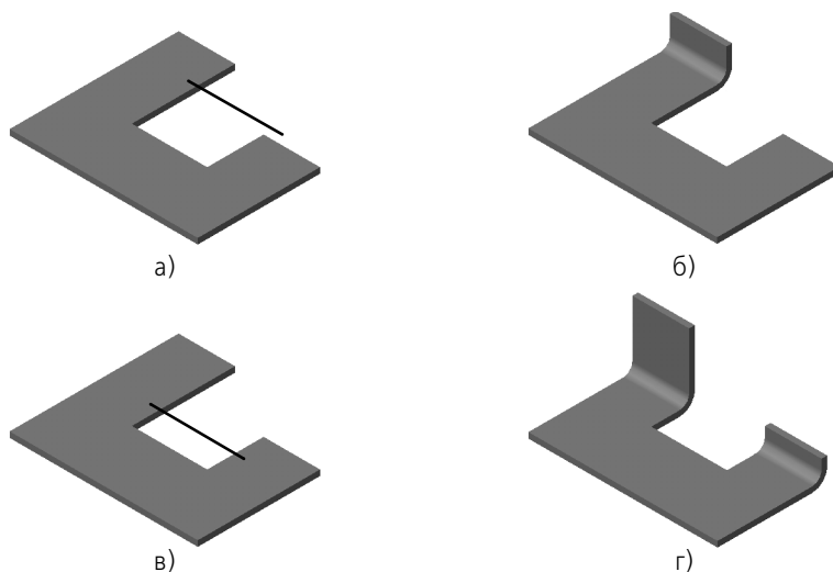
Рис. 97.20. Зависимость результата сгиба от положения линии сгиба: а), в) варианты положения линии сгиба, б), г) соответствующие результаты построения
