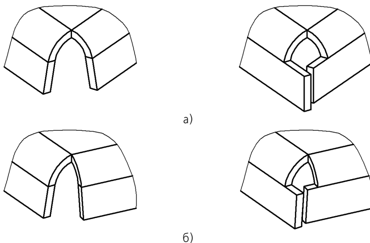
Рис. 97.37. Замыкание с перекрытием (исходное состояние детали и результат операции): а) замыкаемый угол острый, б) замыкаемый угол тупой
